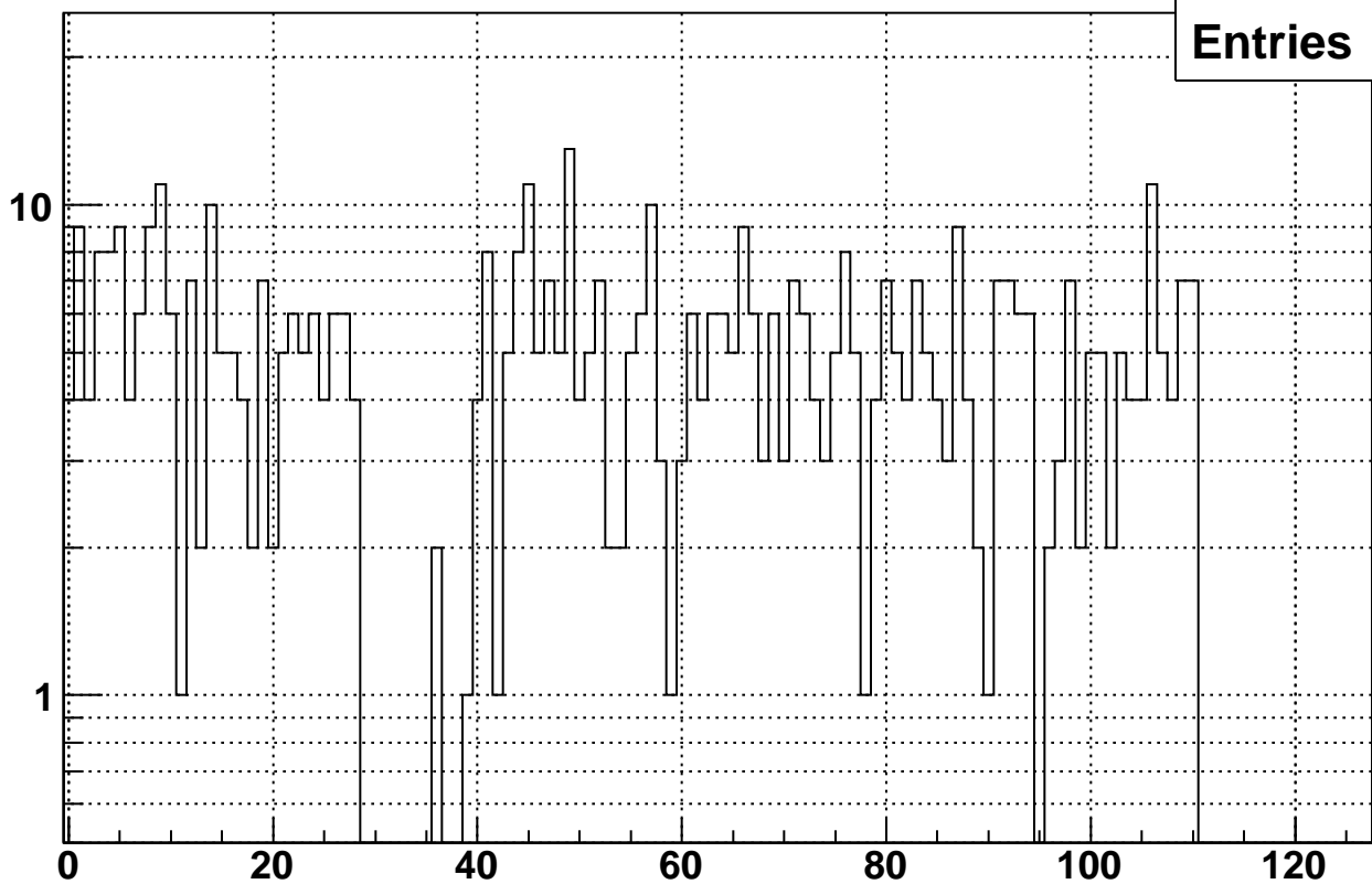
Rate vs. raw bx7 Fill 10476
