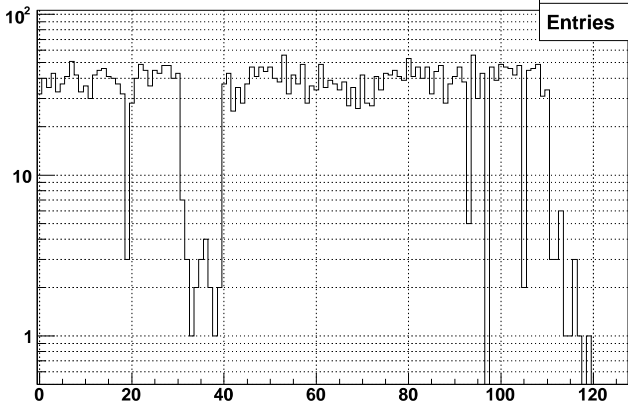
Rate vs. raw bx7 Fill 10449
