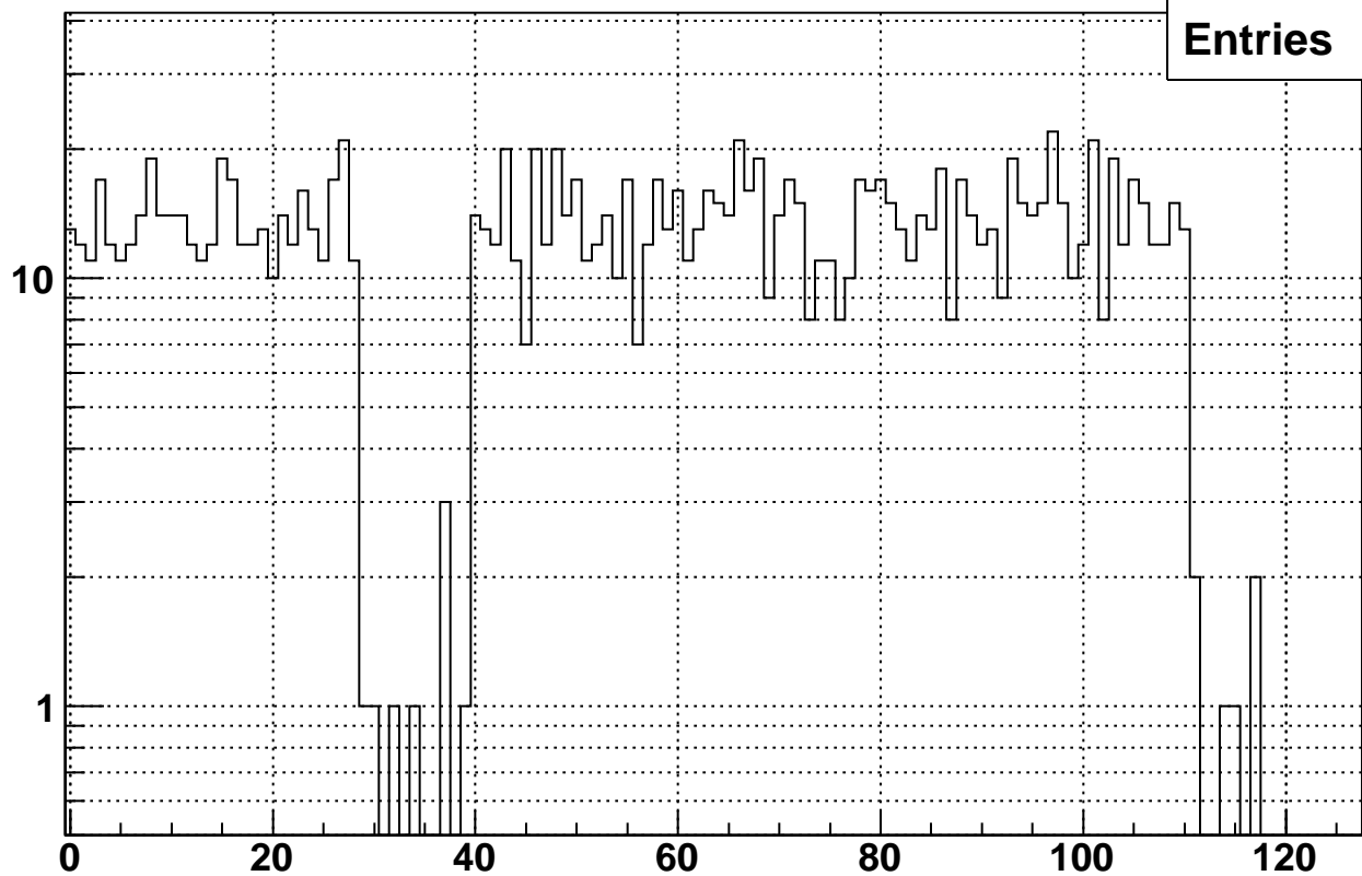
Rate vs. raw bx7 Fill 10528
