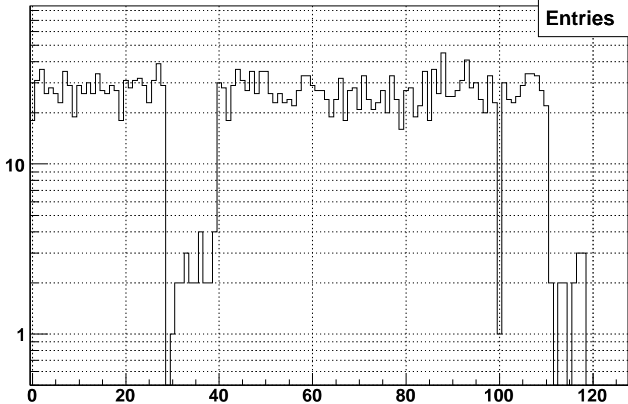
Rate vs. raw bx7 Fill 10486
