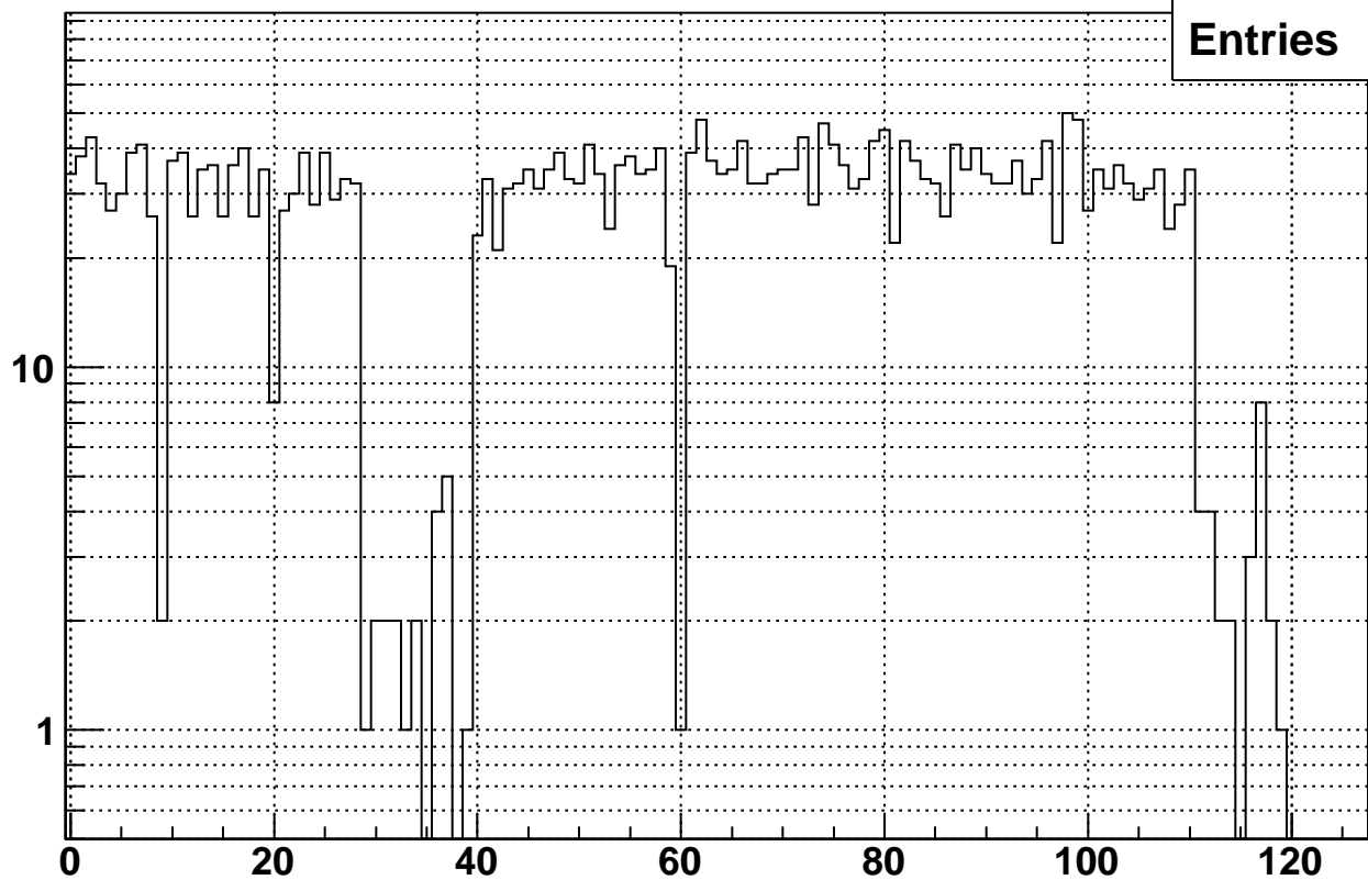
Rate vs. raw bx7 Fill 10490
