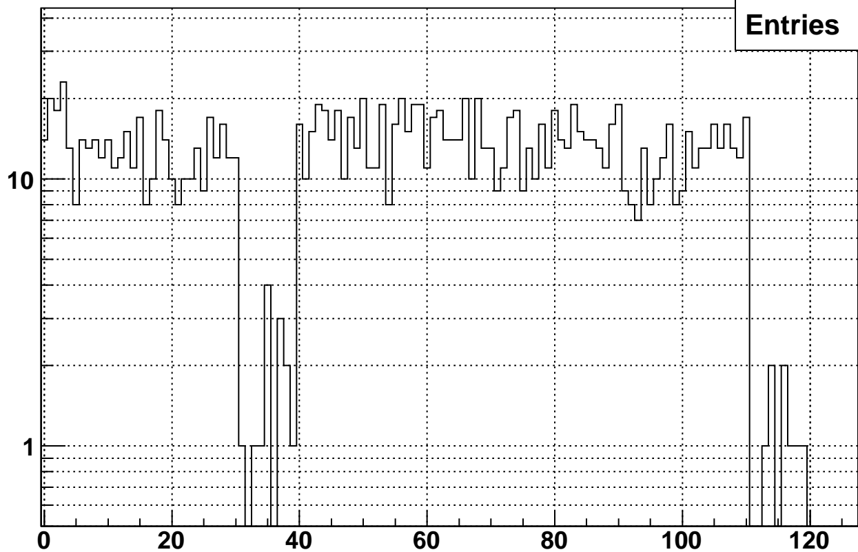
Rate vs. raw bx7 Fill 10407
