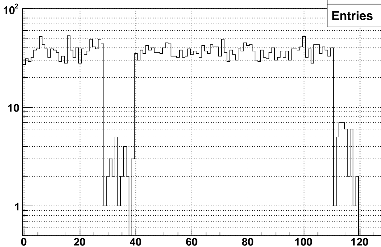
Rate vs. raw bx7 Fill 10525
