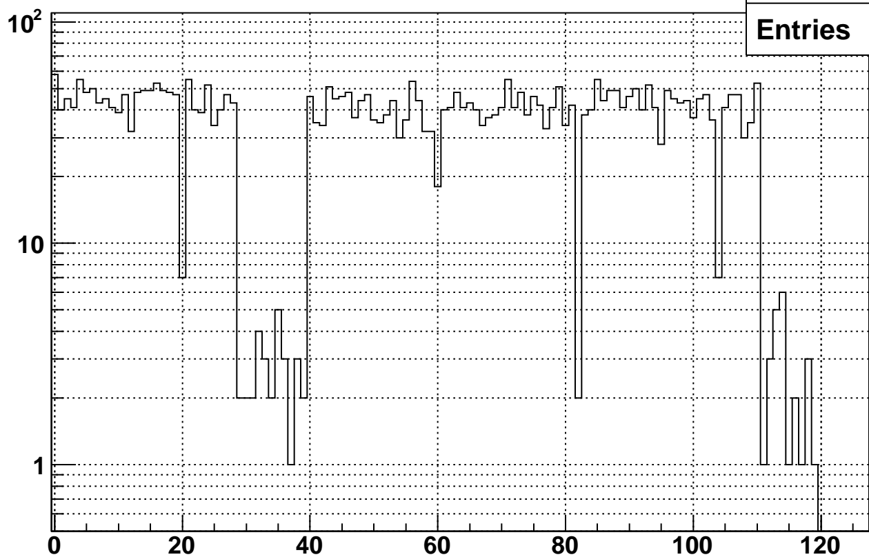
Rate vs. raw bx7 Fill 10535
