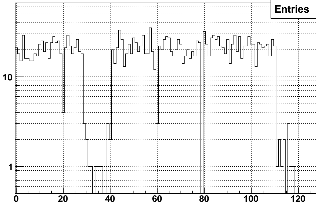
Rate vs. raw bx7 Fill 10482
