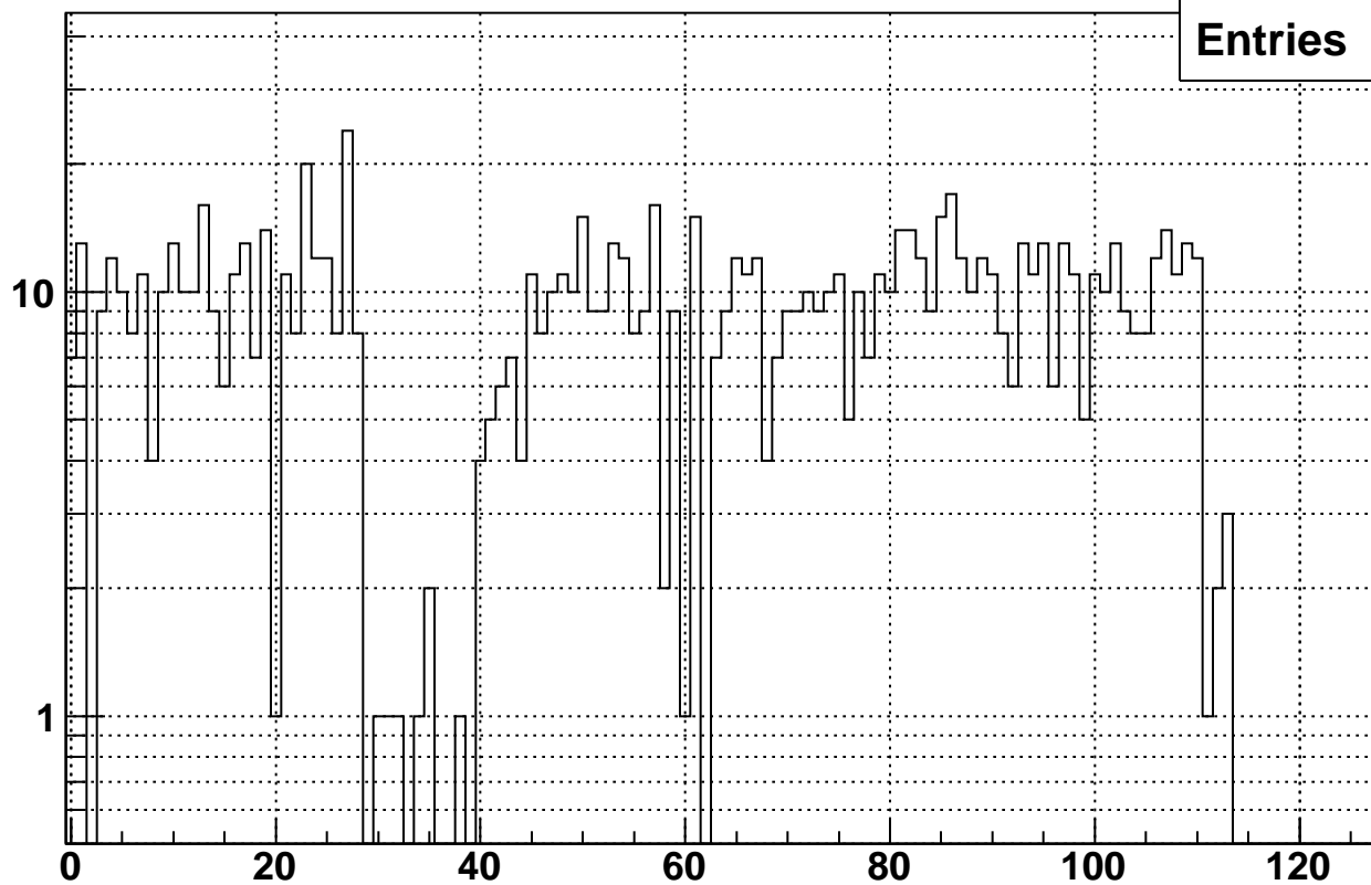
Rate vs. raw bx7 Fill 10508
