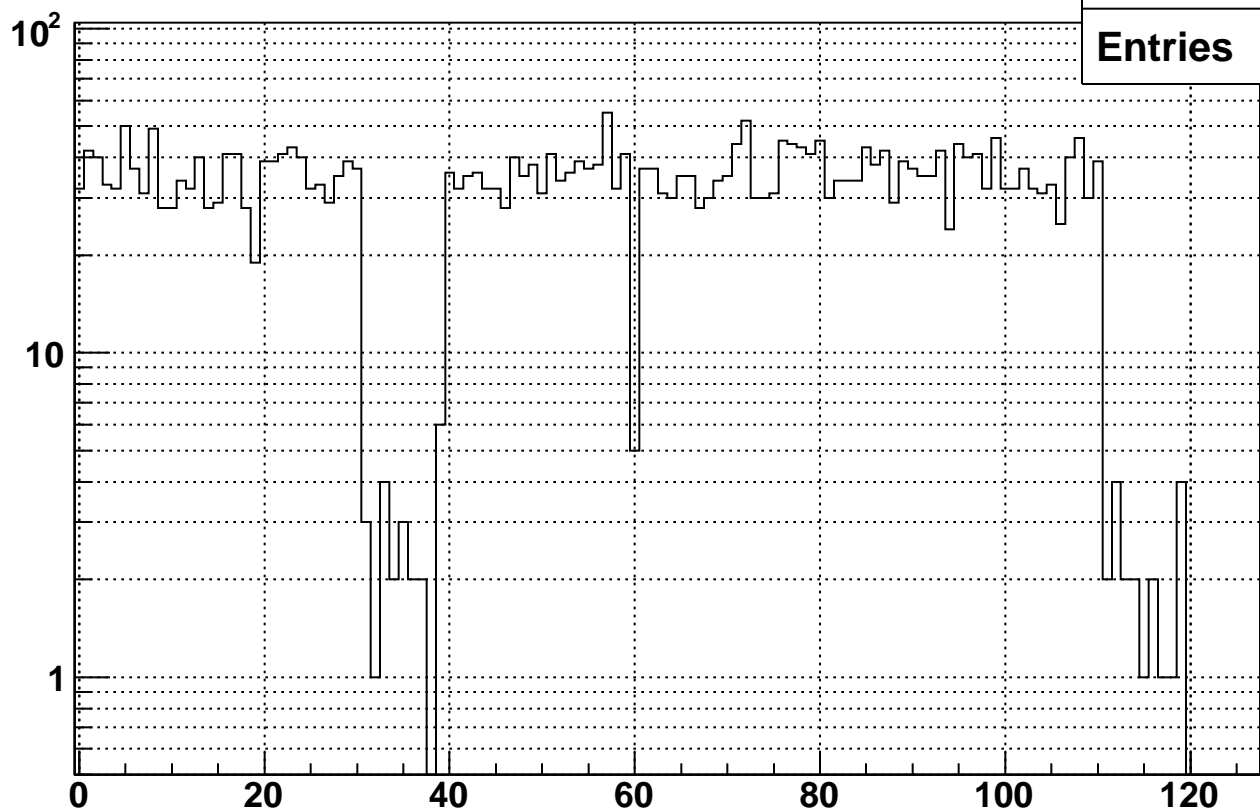
Rate vs. raw bx7 Fill 10448
