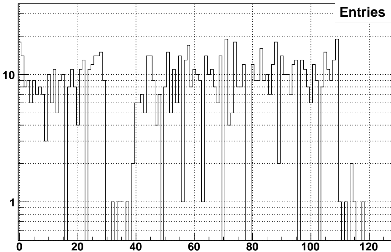
Rate vs. raw bx7 Fill 10402
