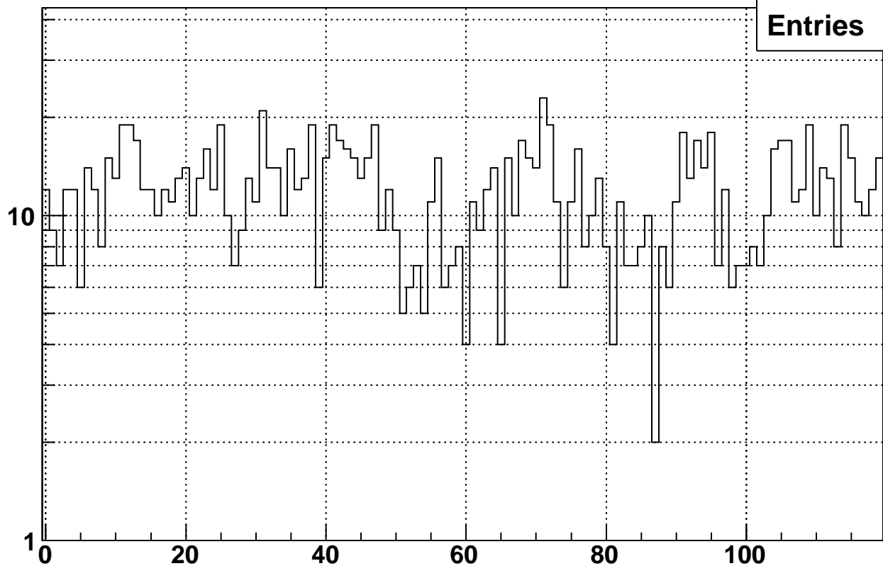
Rate vs. raw bx48 Fill 10407
