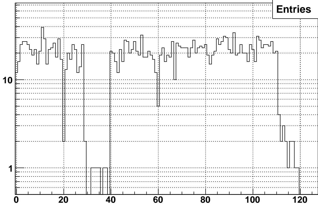
Rate vs. raw bx7 Fill 10526
