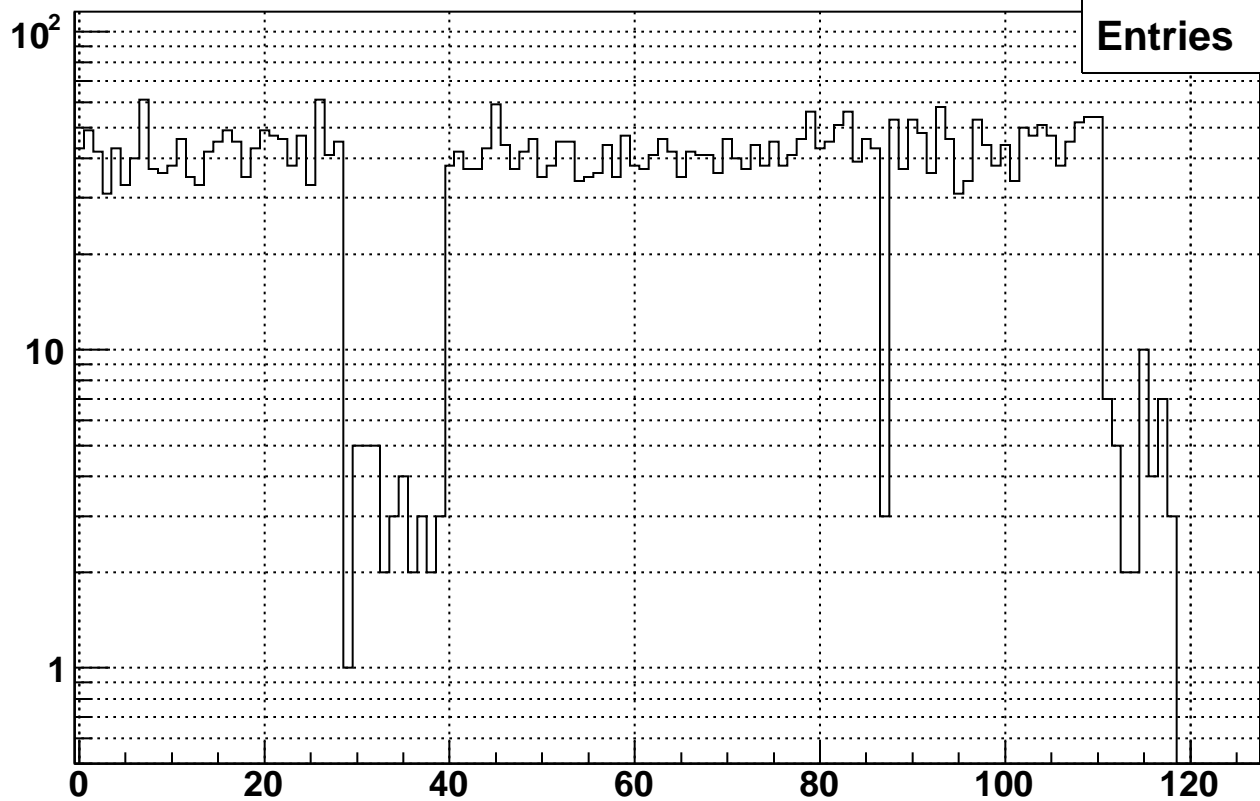
Rate vs. raw bx7 Fill 10471
