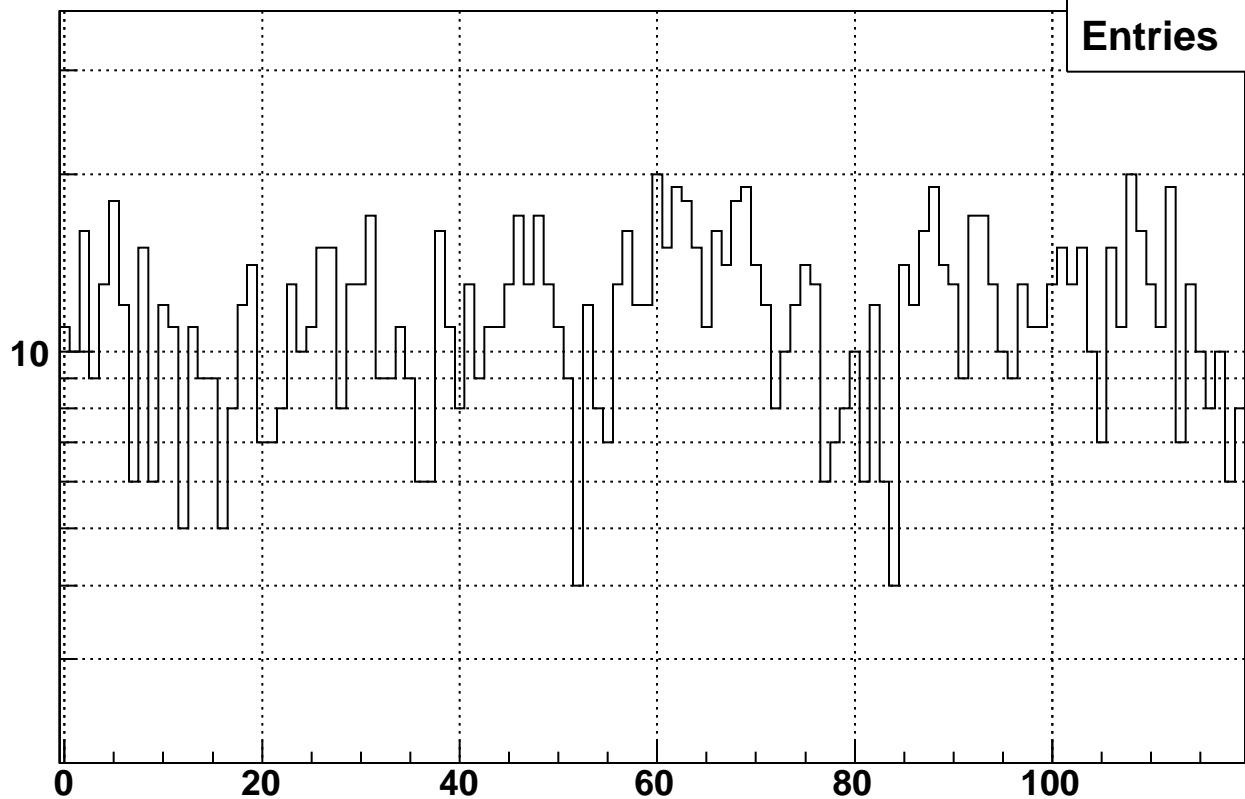
Rate vs. raw bx48 Fill 10528
