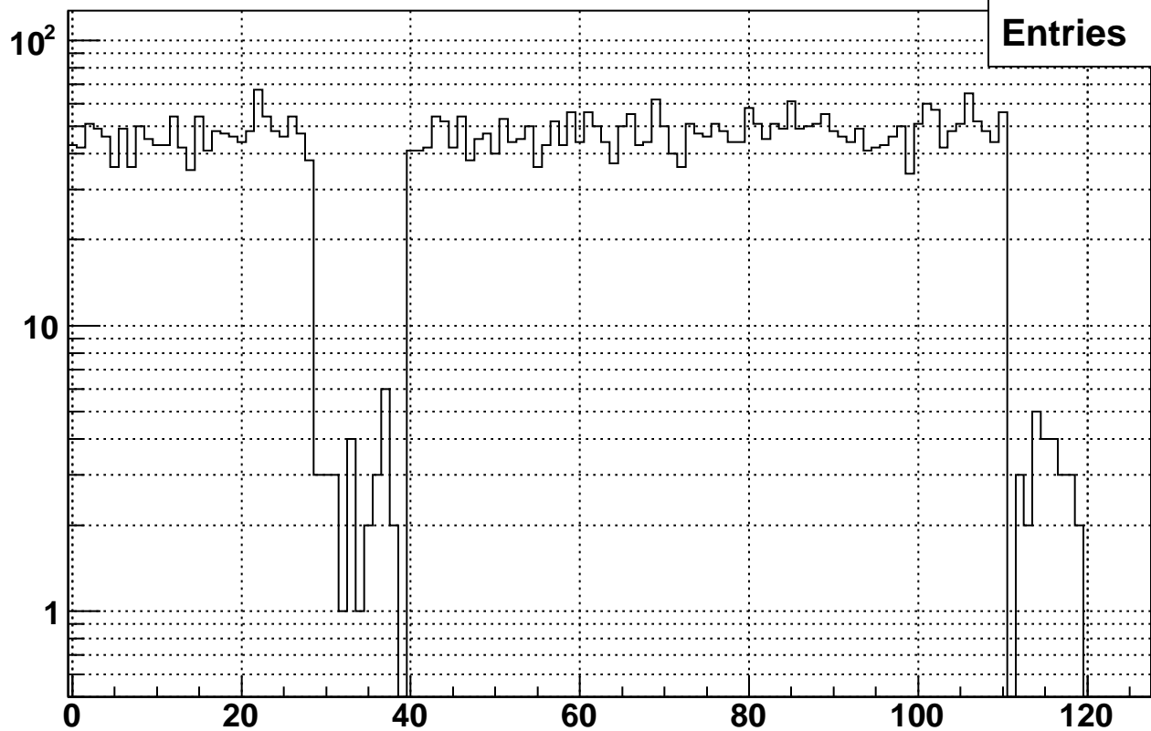
Rate vs. raw bx7 Fill 10531
