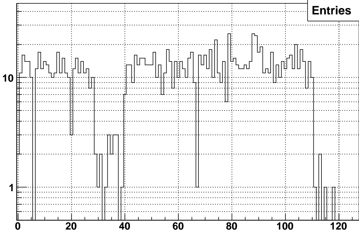
Rate vs. raw bx7 Fill 10536
