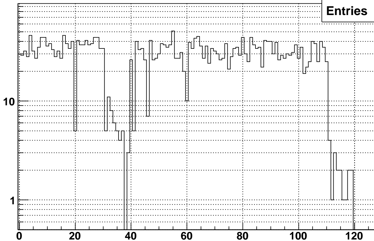
Rate vs. raw bx7 Fill 10450
