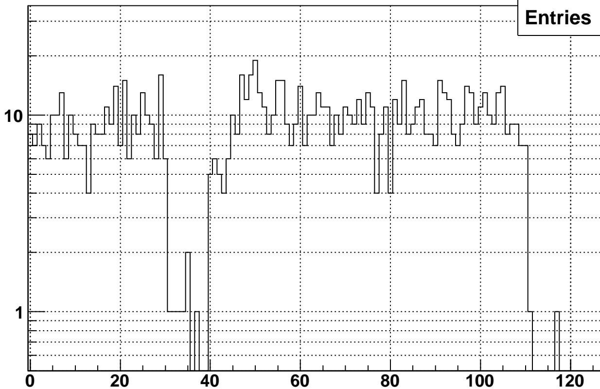
Rate vs. raw bx7 Fill 10426
